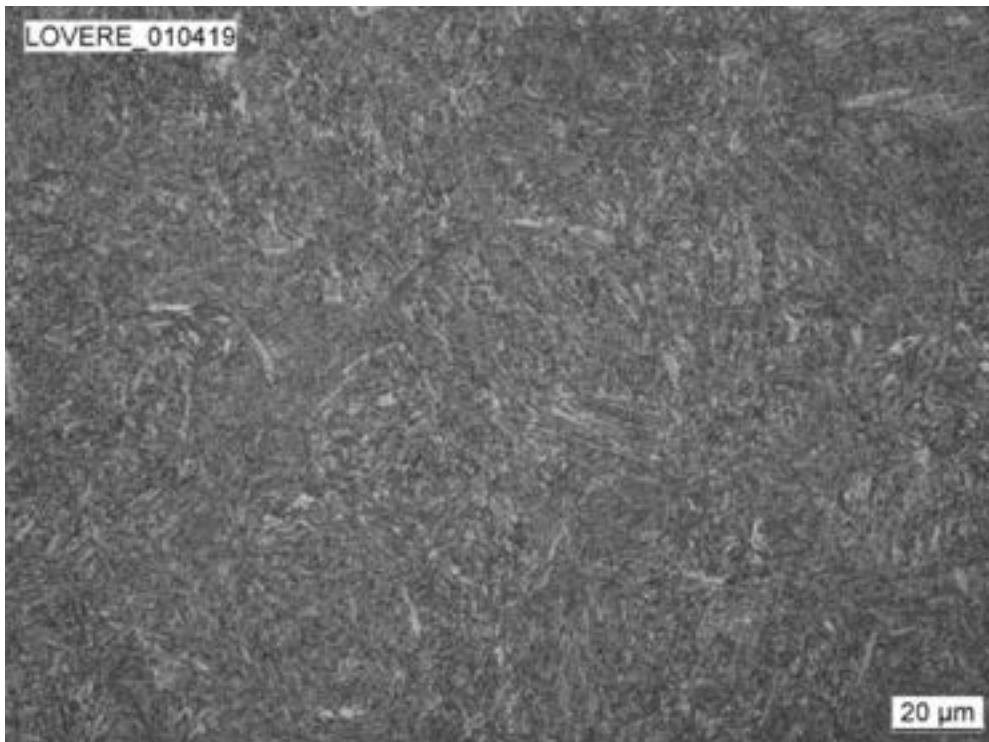
A microestrutura do KeyLos ® UP detetada a cerca de 20 mm abaixo da superfície é martensite revenida.
