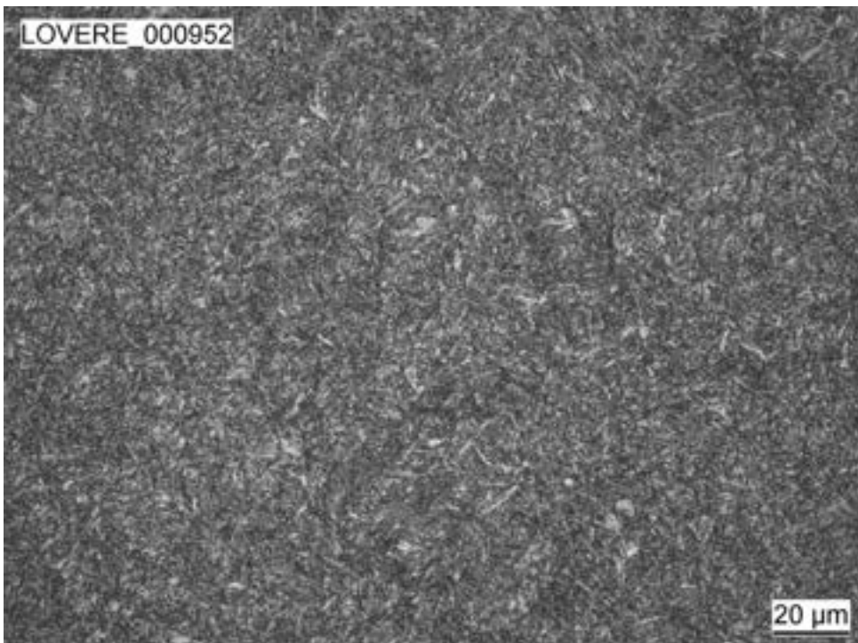
A microestrutura do KeyLos ® 2738 detetada a cerca de 20 mm abaixo da superfície é martensite revenida
