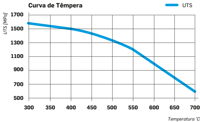
A curva de têmpera de uma amostra que foi austenizada a 850 °C
