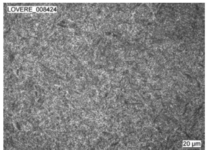
A microestrutura do KeyLos ® 2311 detetada a cerca de 20 mm abaixo da superfície é martensite revenida.
